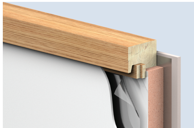
Geeignet für kompakte und energiesparende Holzrahmbau bei Neubau und Sanierung nach EnEV. Die Landesbauordnungen sind zu beachten.
